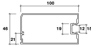
VERTICAL DOOR
