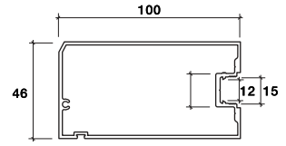
VERTICAL DOOR
