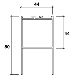
BOTTOM DOOR
