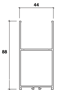
BOTTOM DOOR
