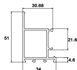
TOP DOOR
