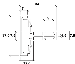
HORIZONTAL DOOR
