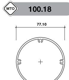
POLE
