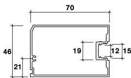
VERTICAL DOOR
