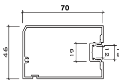
VERTICAL DOOR
