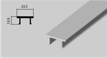
► LT.09 Flush Stop
