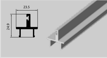
► LT.08 45 mm. Door Stop
