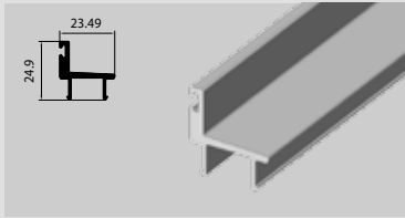
► LT.07 35 mm. Door Stop
