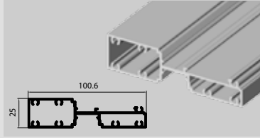
► LT.15 Horizontal Mid rail
