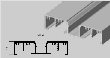
► LT.02 100 mm. Mullion
