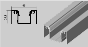
► LT.45-02 45 mm. Mullion
