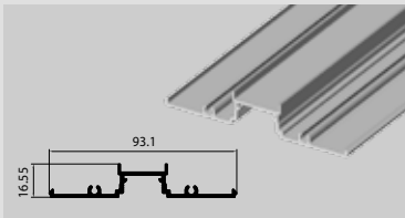
► LT.04 100 mm. Snap Mullion
